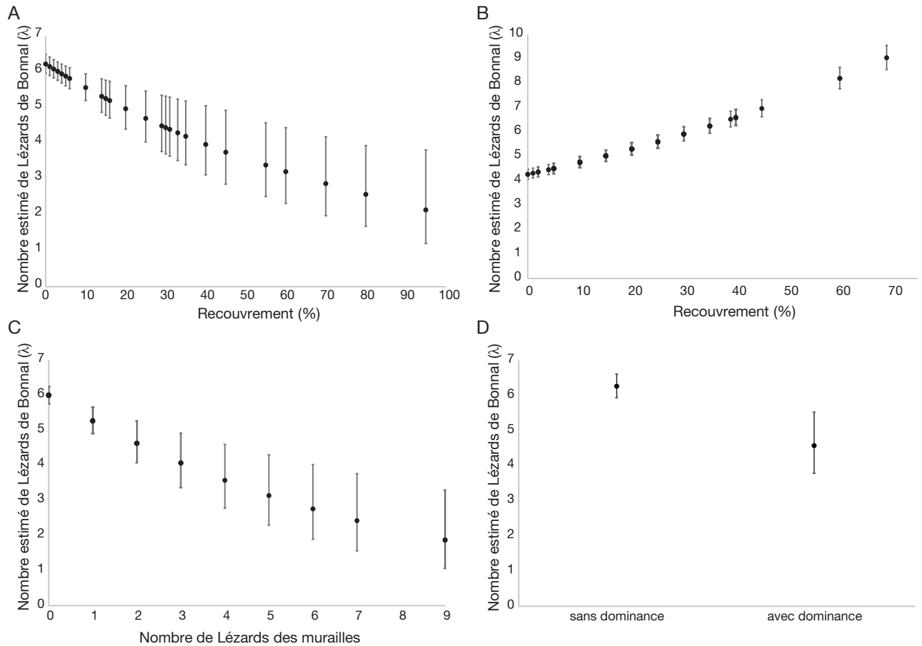
FIG. 7. — Nombre estimé de Lézard de Bonnal Iberolacerta bonnali (Lantz, 1927) (A) par une méthode des N-mixture (distribution de Poisson) en fonction des principales covariables : A , recouvrement de gros bloc ; B , recouvrement de la strate herbacée ; C , nombre relatif de Lézards des murailles ; D , dominance de la roche granitique. Moustaches = intervalles de confiance bayésiens à 95 %.
