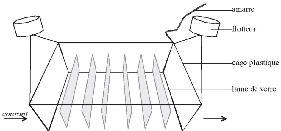
Fig. 2. Représentation schématique d'un dispositif utilisé pour la collecte du périphyton. Schematic representation of one rack of artificial substrates used for algal attachment.
