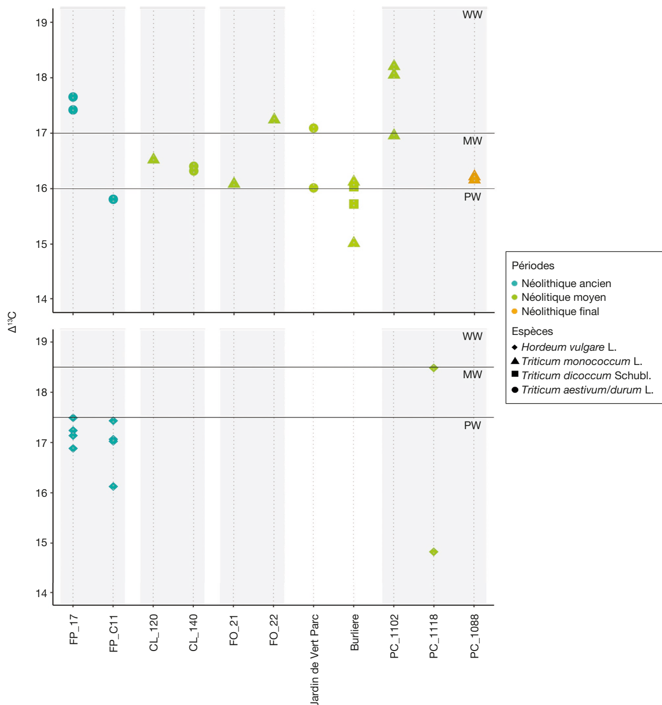
Fig. 2. — Valeurs isotopiques de \Delta^{13}\text{C} et disponibilité en eau. Sites : CL_120, CL_140, Claparouse; FO_21, FO_22, Fontbrégoua; FP_17, FP_C11, la Font-aux-Pigeons; PC_1102, PC_111, PC_1088, la Perte du Cros. Abréviations : MW, apport en eau modéré; PW, apport en eau insuffisant ou faible; WW, bon apport en eau.
