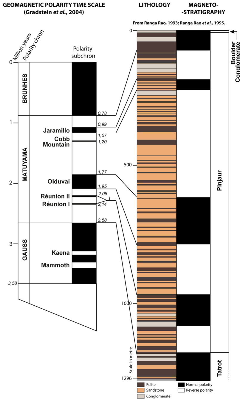
Fig. 2. Magnetostratigraphy of the Patiali Rao section from Ranga Rao (1993) and Ranga Rao et al. (1995). Fig. 2. Magnétostratigraphie de la séquence stratigraphique du Patiali Rao d'après Ranga Rao (1993) et Ranga Rao et al. (1995).
