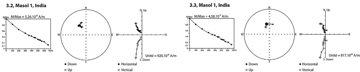
Fig. 9. Thermal demagnetization for the two Masol Unit C samples (PPM4 block): change of the magnetization, stereographic projection, Zijderveld diagram. Fig. 9. Désaimantation thermique des deux échantillons de l'unité C (PPM4 block) : désaimantation, projections stéréographiques, diagramme de Zijderveld.
