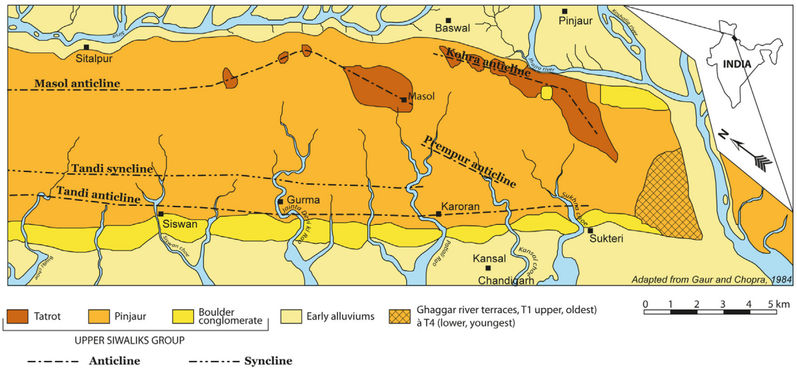
Fig. 1. Geological map of the Chandigarh anticline in the Siwalik Frontal Range. Fig. 1. Carte géologique de l'anticlinal de Chandigarh dans la chaîne frontale des Siwaliks. Adapted from Gaur and Chopra (1984).
