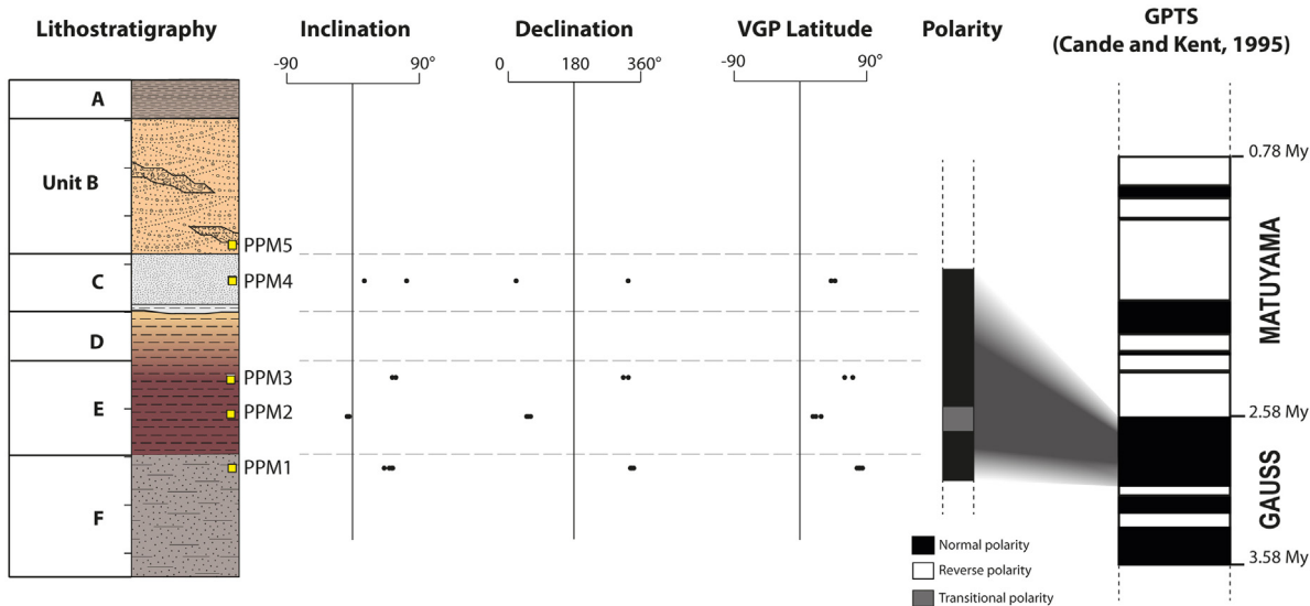
Fig. 10. Lithostratigraphy and magnetostratigraphy of the Masol 1 section. Fig. 10. Lithostratigraphie et magnétostratigraphie de la coupe de Masol 1.
