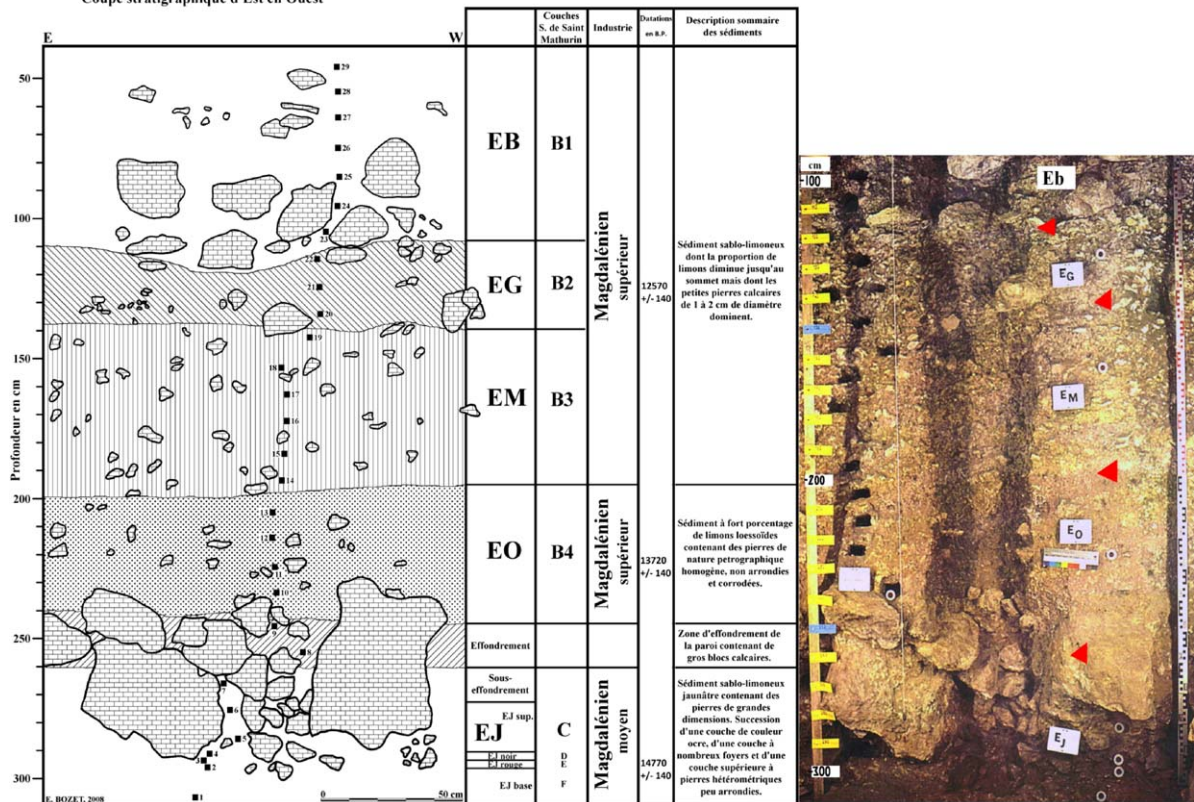
Fig. 2. Coupe stratigraphique d'est en ouest du Roc-aux-Sorciers (Angles sur l'Anglin, Vienne). Les noms attribués aux différentes couches de sédiments utilisés dans la description stratigraphique sont corrélés aux couches archéologiques définies par Saint-Mathurin et Garrod lors de leurs fouilles. La coupe de 310 cm d'épaisseur montre trois niveaux d'occupations : Magdalénien moyen, début du Magdalénien supérieur et Magdalénien supérieur. Les prélèvements sédimentologiques ont été réalisés sur l'ensemble de la coupe en continuité.
