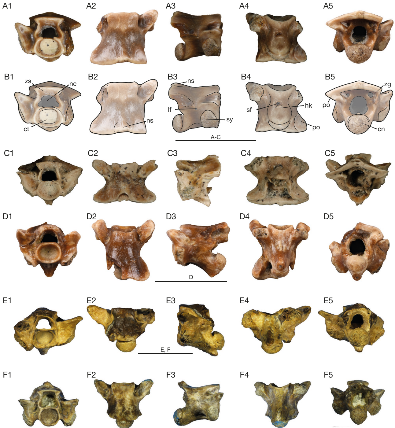
FIG. 3. — Colombophis portai Hoffstetter & Rage, 1977 specimens! A, B, VPPLT-1006; C, VPPLT-0067; D, VPPLT-0068; E, VPPLT-1739; F, VPPLT-1735. Views: 1, anterior; 2, dorsal; 3, lateral; 4, ventral, 5, posterior views. Scale bars: 10 mm.
